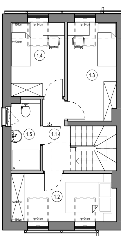
PODDASZE
