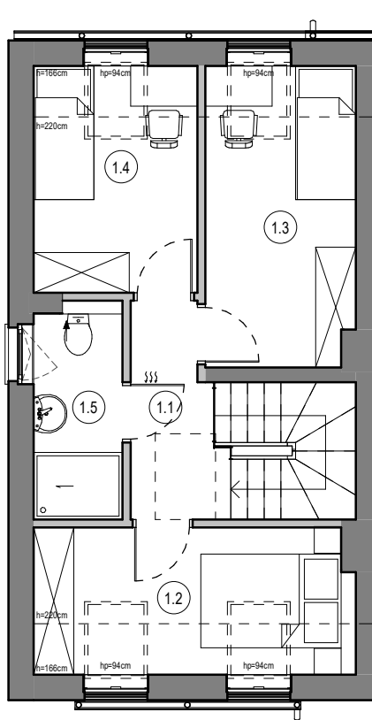
PODDASZE
